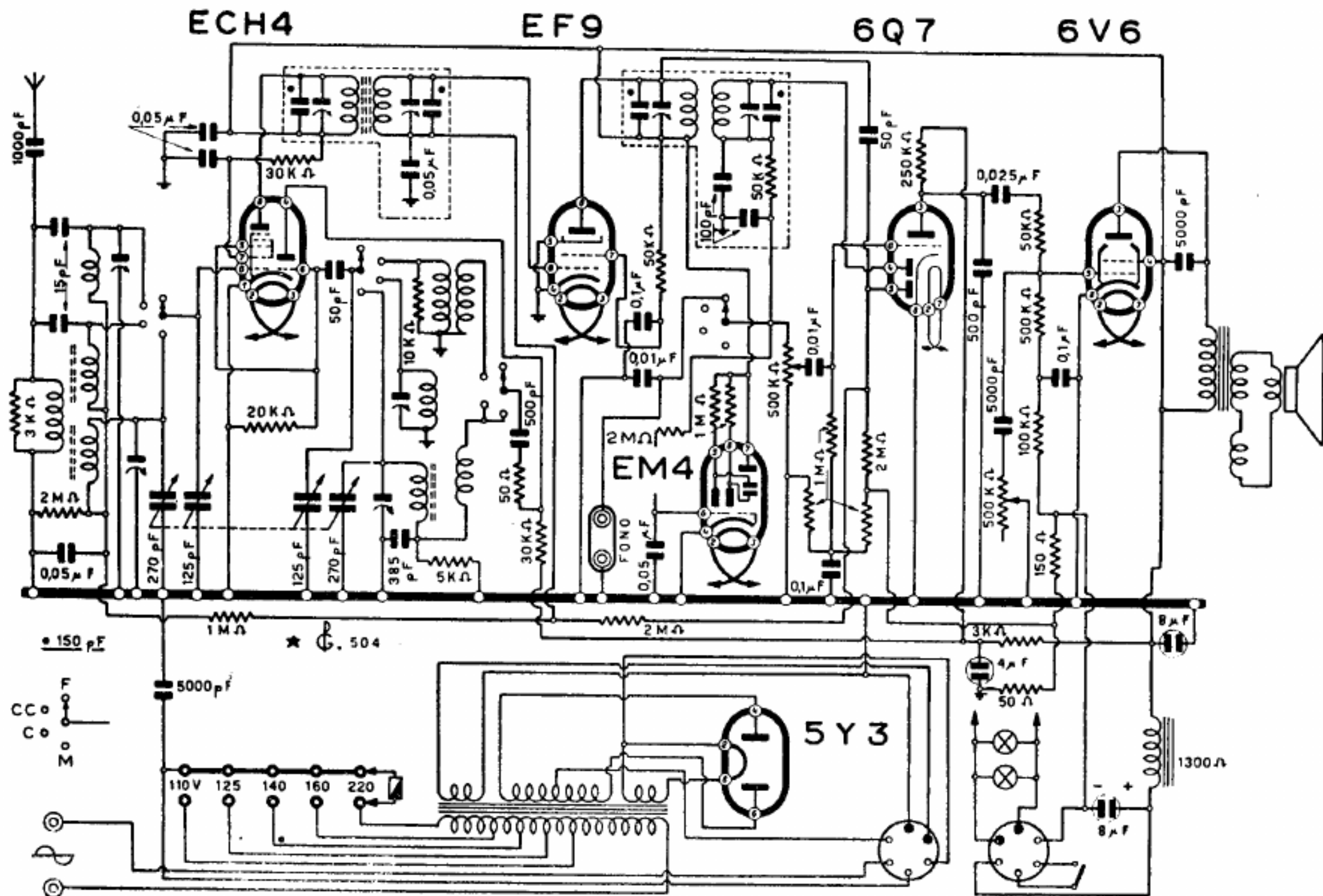
Lo schema elettrico del mod. Umbria (valore della MF 465 kHz)
